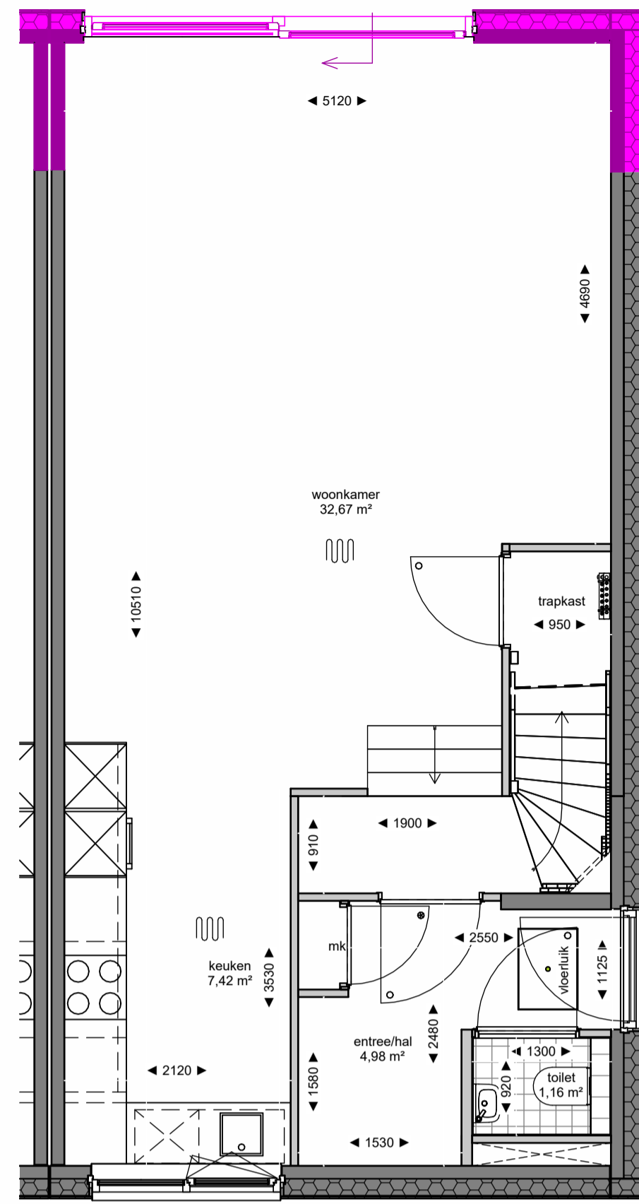
Begane grond
