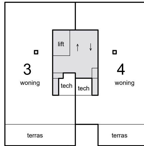
1e verdieping
